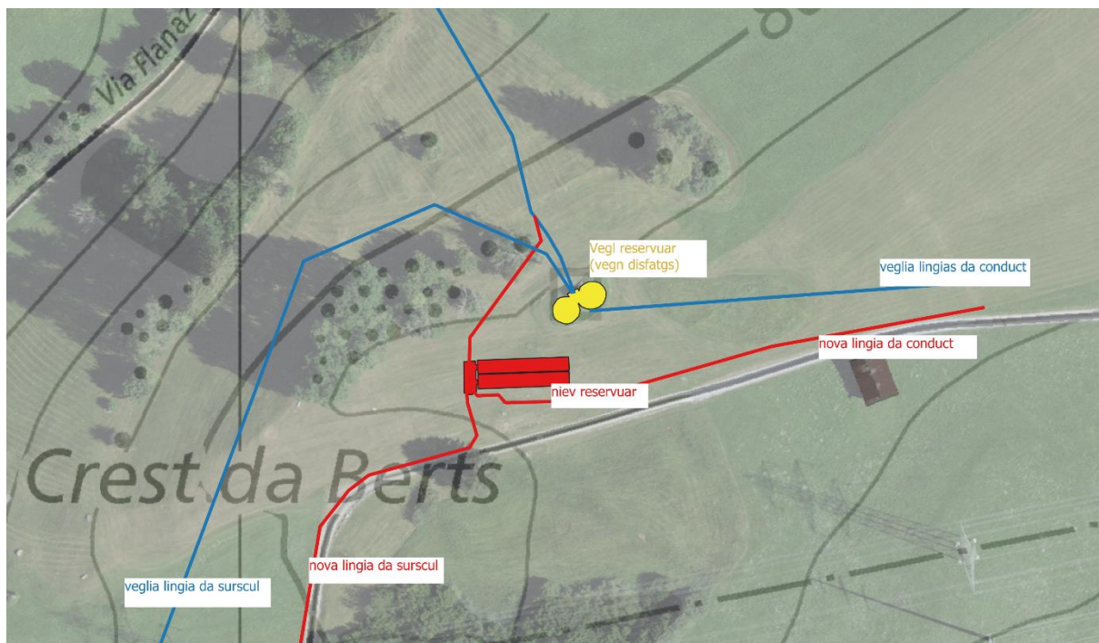
Maletg 1: Plan da situaziun
