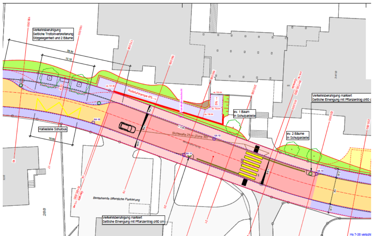
Abbildung 2: Ausgestaltung mit Rampe im Bereich des Schulhauses.
