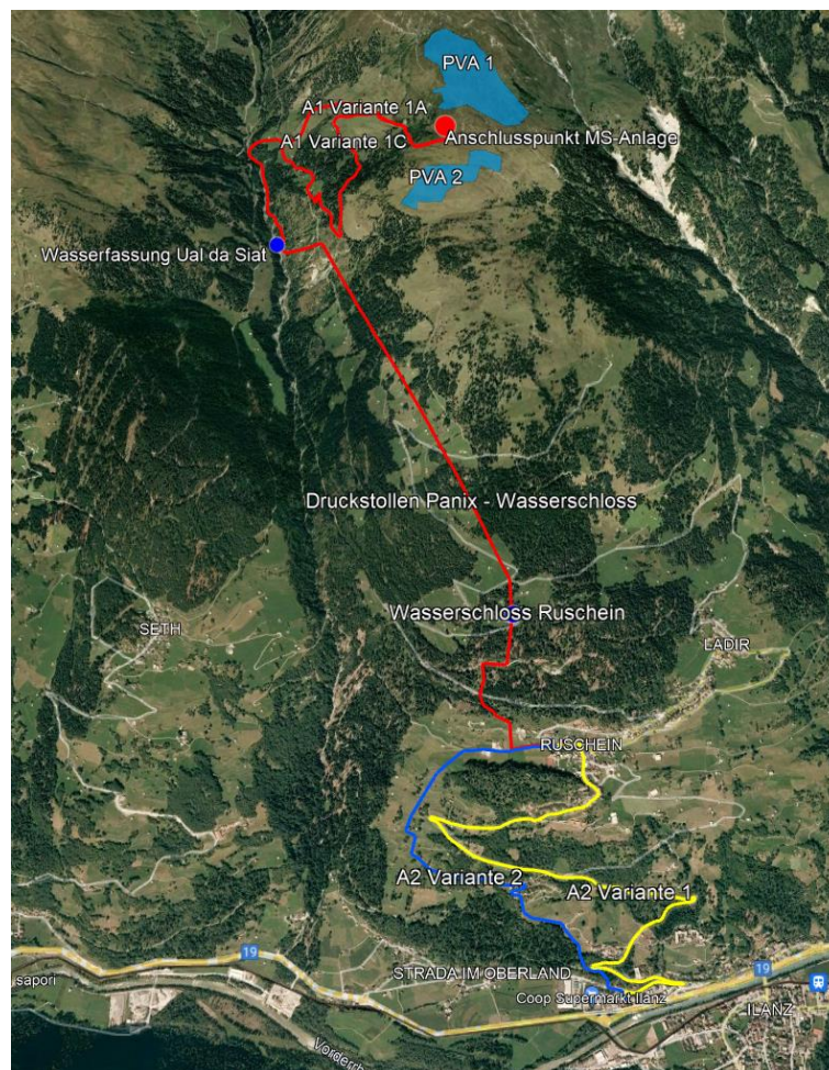
Abbildung 3: Anschlussleitung
